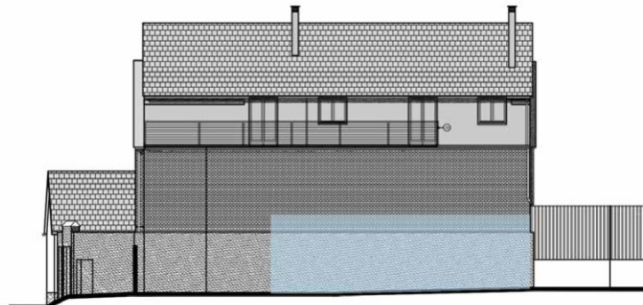
Pohled západní
