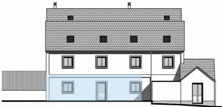
Pohled východní
