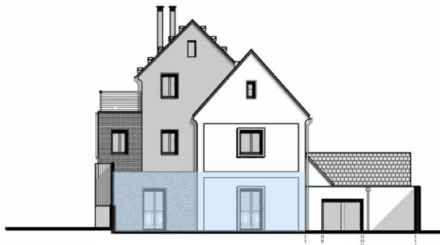
Pohled jižní
